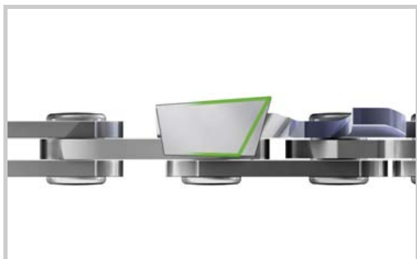
Angolo di affilatura troppo ottuso
