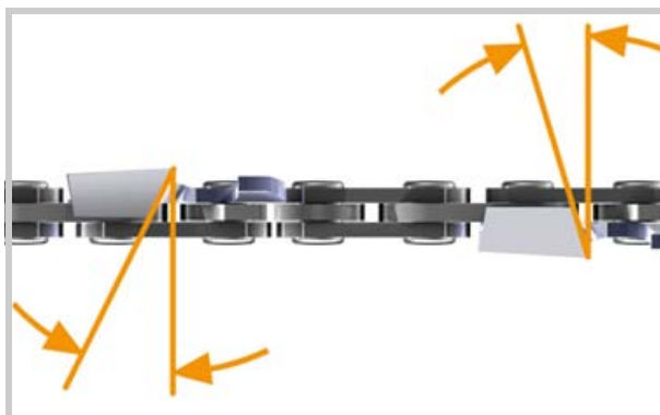
Angoli di affilatura diversi
