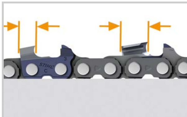
Lunghezze di dente diverse
