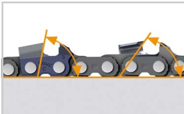
Angoli del tagliente laterale diversi
