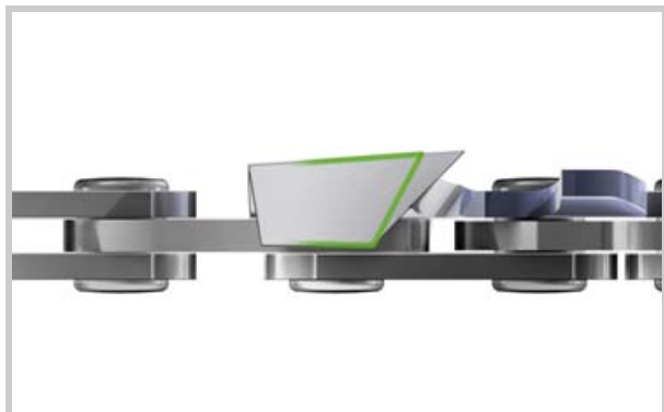
Angolo di affilatura troppo acuto
