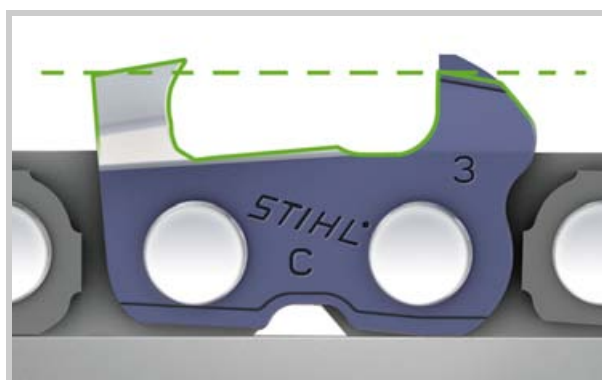
Limitatore di profondità troppo alto
