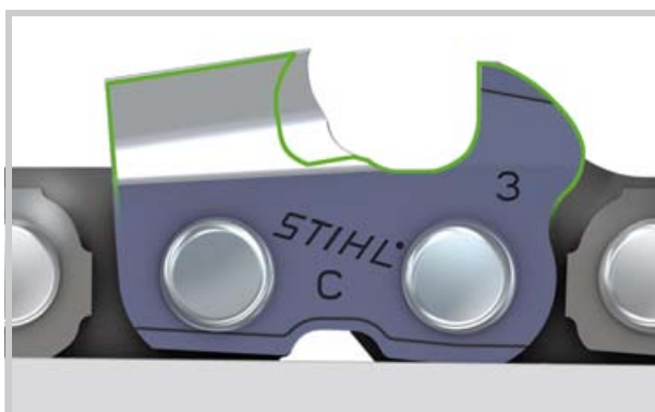
Angolo del tagliente laterale all'indietro
