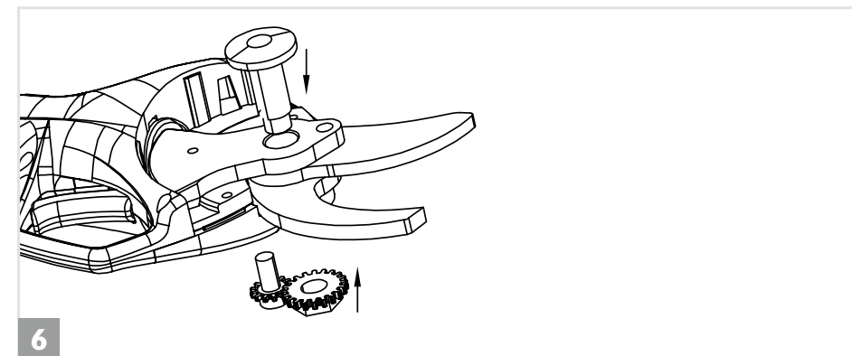
6. Zahnradmutter und Einstellclip festziehen.
